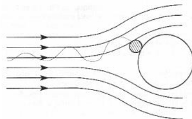
Figure 8 : Mécanismes de capture des particules sur une fibre – Effet de diffusion
